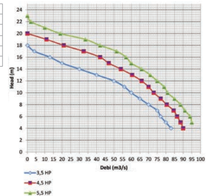
Debi Diyagramı
